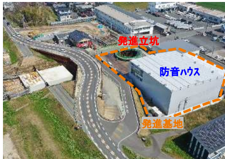
発進基地状況 (防音ハウス組立状況)
